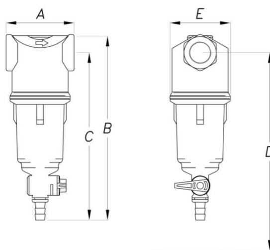
Bravo senza manometro cod. FT300, FT302, FT304
